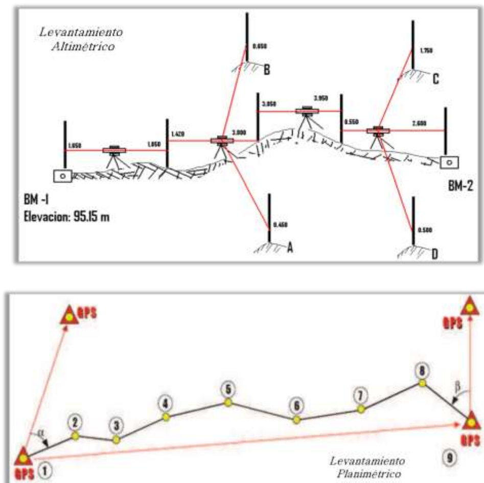
Figura 2. Esquemas de Ejemplo de Levantamientos Topográficos en Altimetría y Planimetría controlados con puntos geodésicos 2 .
