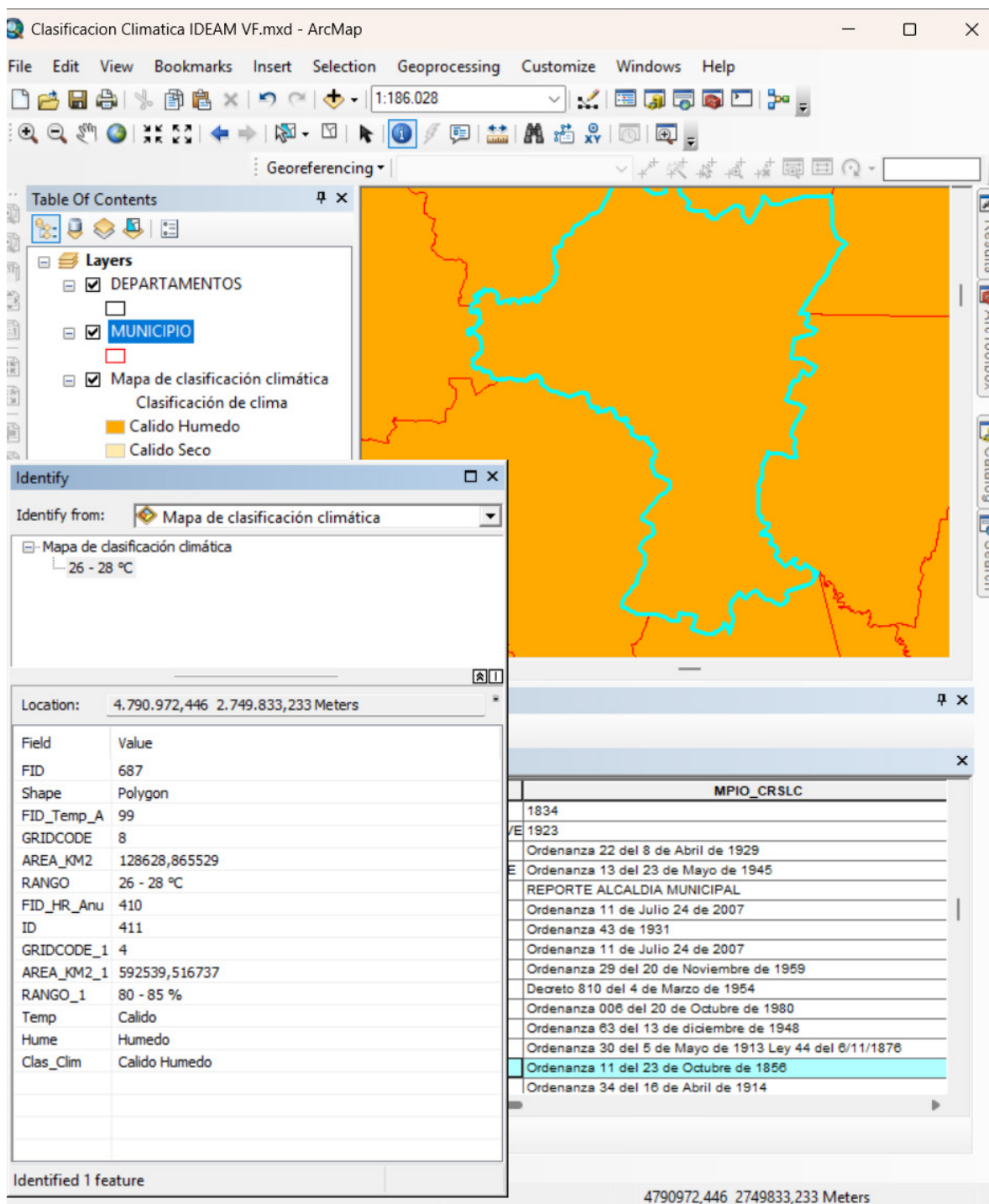
Ilustración 6. Clasificación climática
